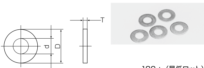
平ワッシャー
