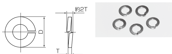
スプリングワッシャー
