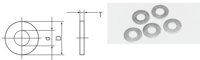
平ワッシャー
