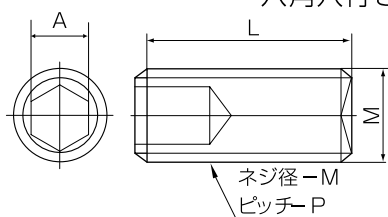
六角穴付き止めネジ クボミ先
