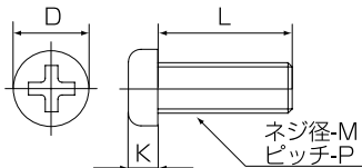
十字穴付ナベコネジ
