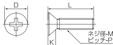
十字穴付サラコネジ
