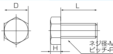
六角ボルト
