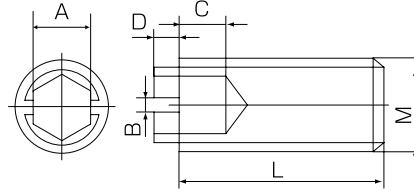
イモネジ
